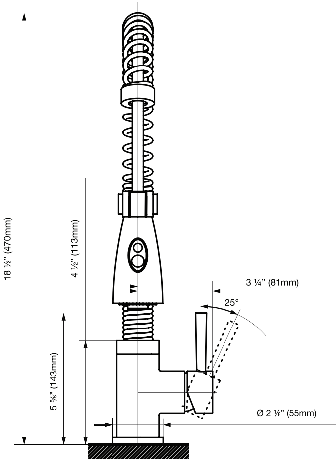
SIDE VIEW / VUE DE CÔTÉ / VISTA LATERAL
