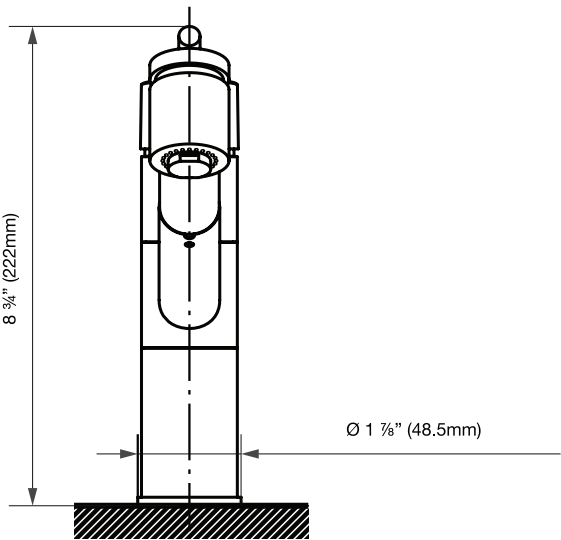
SIDE VIEW / VUE DE CÔTÉ / VISTA LATERAL
