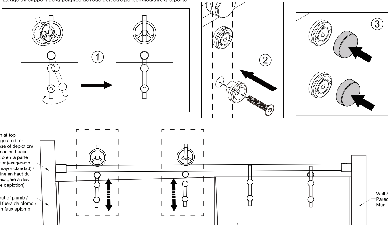
FIG.3 The wheel handle bracket rod must be perpendicular to the door. La varilla del soporte de la manija de la rueda debe estar perpendicular a la puerta. La tige du support de la poignée de roue doit être perpendiculaire à la porte
