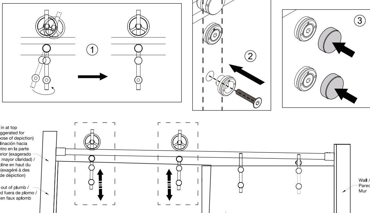
FIG.2 The wheel handle bracket rod must be perpendicular to the door. La varilla del soporte de la manija de la rueda debe estar perpendicular a la puerta. La tige du support de la poignée de roue doit être perpendiculaire à la porte
